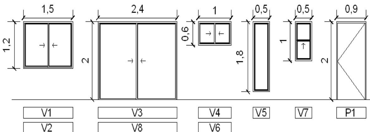
Fig. 2: Carpinterías de la vivienda tipo "Hogares Casas". Representan el 19,56% de la superficie lateral de la envolvente
