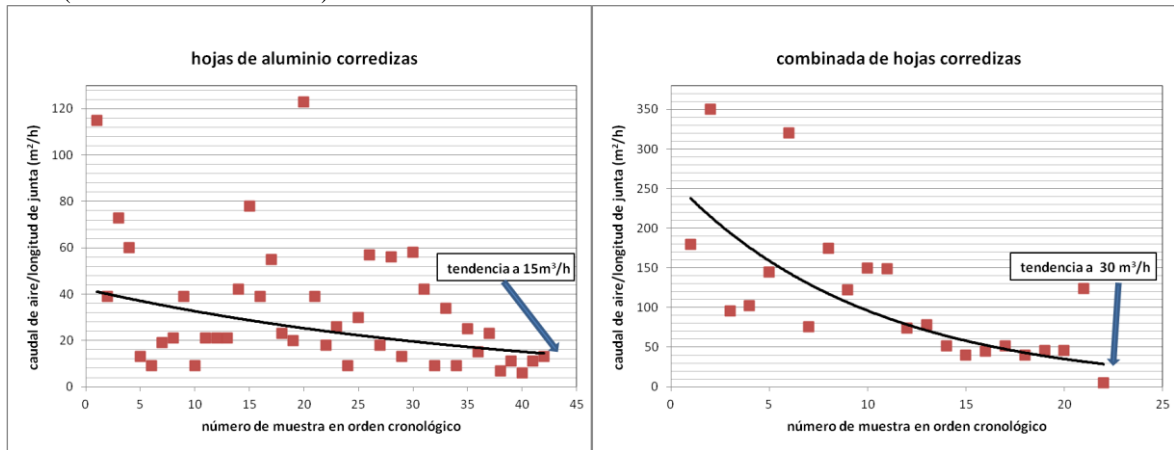
Fig. 3: Tendencia de los caudales de aire infiltrado (m³/h) por m lineal de junta, en dos tipos habituales de carpinterías. Son 42 casos durante el período 1985-2007 para las de aluminio corredizas y 22 casos entre 1985-2005 para las combinadas corredizas.
