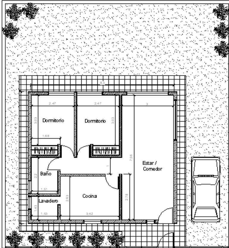
Fig. 1: Planta de vivienda tipo "hogares casa". El modelo es utilizado para la simulación numérica con el programa Energy Plus, a los fines del cálculo de la carga térmica de calefacción anual. El sistema constructivo es de mampostería de ladrillos cerámicos huecos revocados en ambas caras, con el agregado de placas de material aislante térmico. La cubierta es de chapa metálica sobre estructura sostén de madera, con aislación térmica de poliestireno expandido. El modelo cumple con el nivel B de confort higrotérmico de la norma IRAM 11605:2001.
